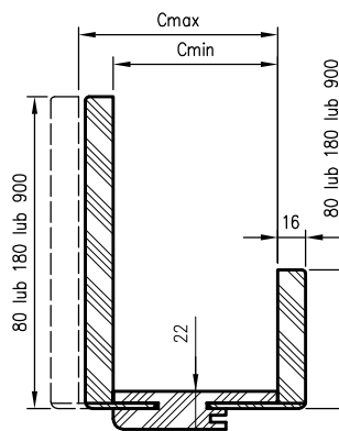
Prierez prekladu ORB maľovaná, spojenie 0°
