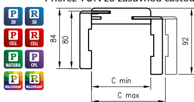
Prierez TUN zo zásuvnou časťou N63
