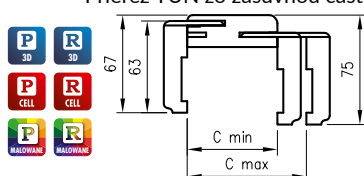
Prierez TUN zo zásuvnou časťou T80
