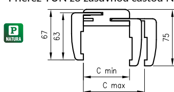
Prierez TUN s uhol. T63
